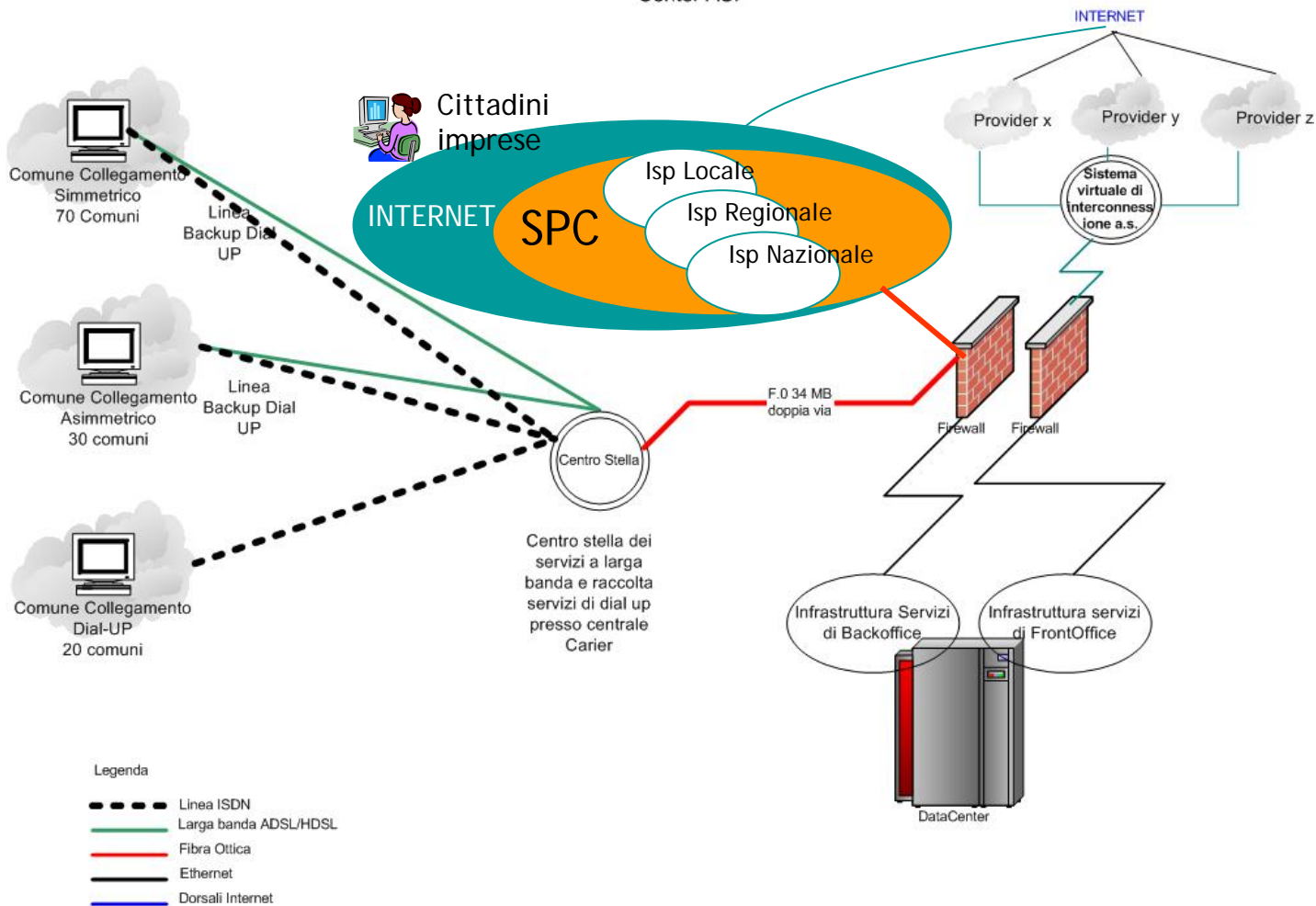
Schema architetturale rete territoriale Data Center ASP
